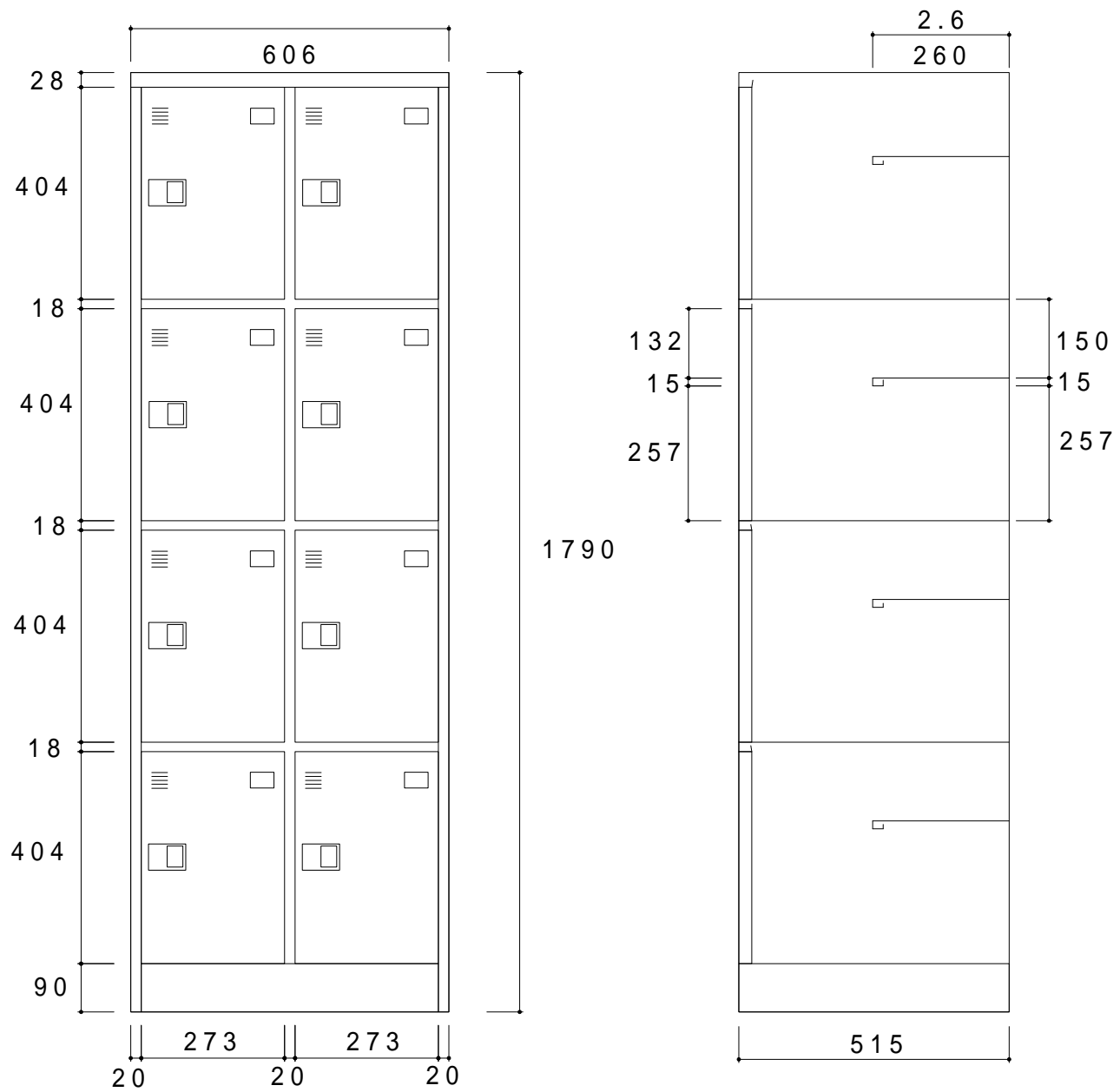
2 列 4 段 W606D515H1790 TNG 中棚 D 260 ( 鋼板 )
